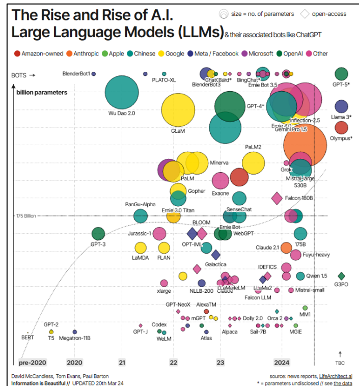
Figura 2: Grans models de llenguatge segons capacitat en milers de milions (bilions US). Els rombes indiquen models de codi obert.
