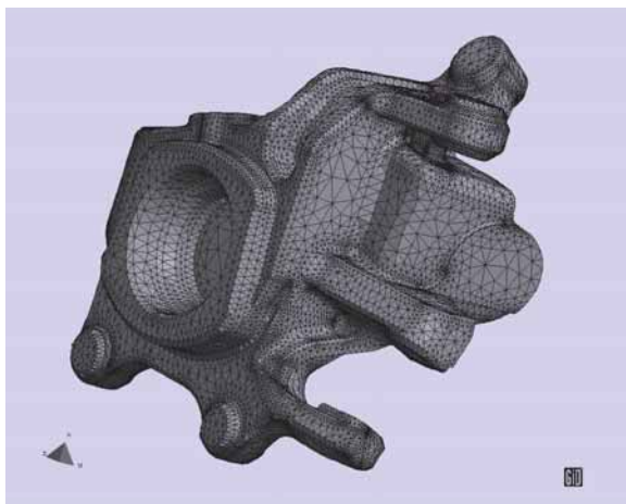
Figura 3 Analisi d'una peça metàl·lica pel mètode dels elements finits
